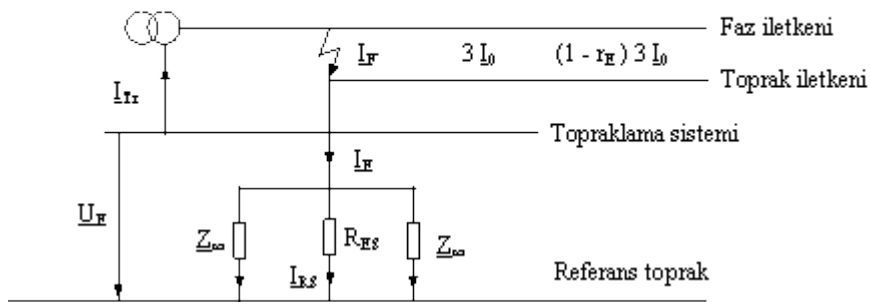
Eşdeğer devre
