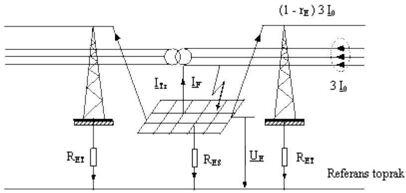
Eşdeğer devre
